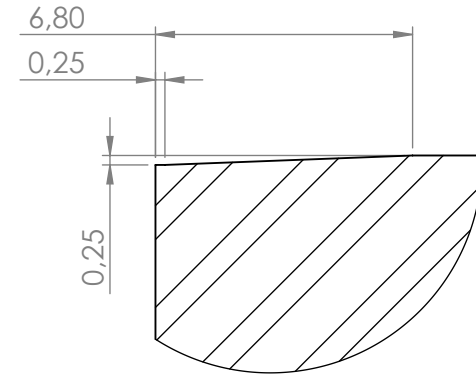
SZCZEGÓŁ B SKALA 5 : 1
