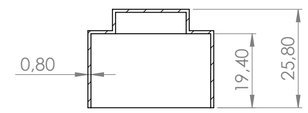
PRZEKRÓJ A-A
