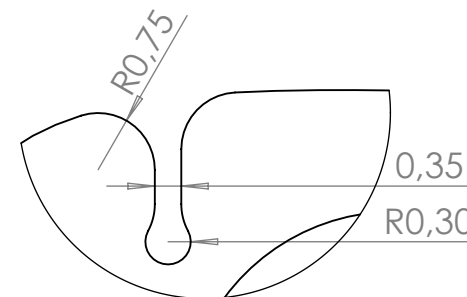
SZCZEGÓŁ A SKALA 10 : 1
